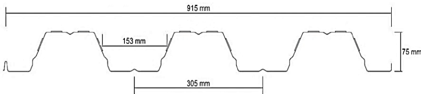
شکل ۲-۹ نمونه‌ای از هندسه یک عرشه فولادی با ارتفاع ۷۵ میلی‌متر
