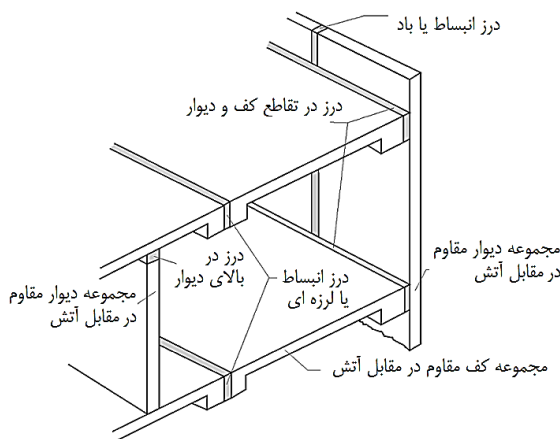
شکل ۷-۱۱ محل‌های معمول قرارگیری درزها
