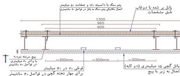
شکل ۲-۳۳ جزئیات اجرای عایق پشم سنگ و گچ برک در زیر سقف
