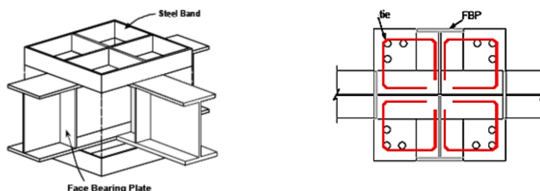
شکل ۱-۳۳ نمونه اتصال RCS دامنه کاربرد و محدودیت‌ها
