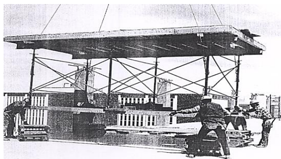
شکل ۱-۵۷ قالب میز پرنده با پایه‌های مهار شده
