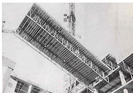
شکل ۱-۵۴ نمونه‌هایی از قالب میزپرنده در حال انتقال
