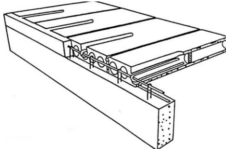
شکل ۱-۲۹ اتصال سقف پیش‌ساخته Hollow Core به تیر نیمه پیش‌ساخته
