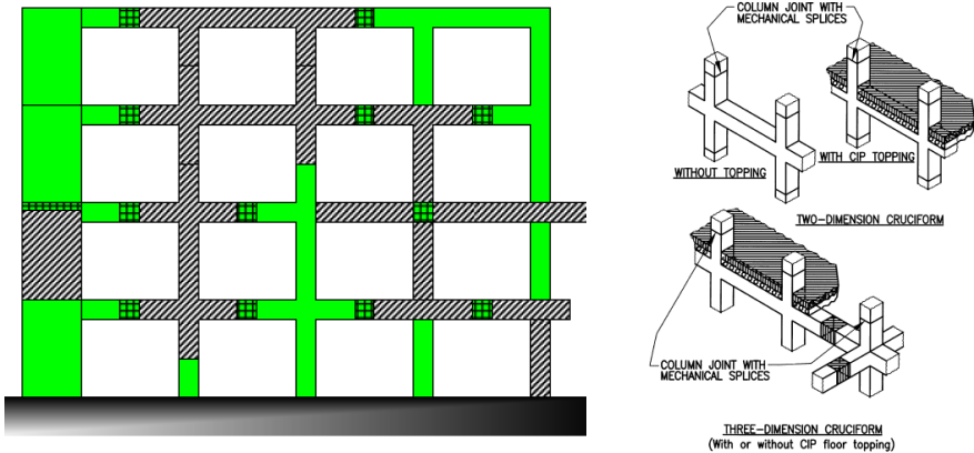
شکل ۱-۲۲ نمونه‌هایی از قطعات دو بعدی و سه بعدی پرتال برای اجرای قاب‌های بتن مسلح پیش‌ساخته
