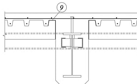
شکل ۲-۱۵ قالب انتهایی
