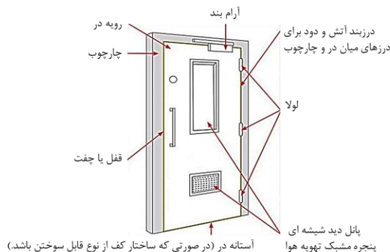
شکل ۴-۷ اجزای تشکیل دهنده در مقاوم در برابر آتش
