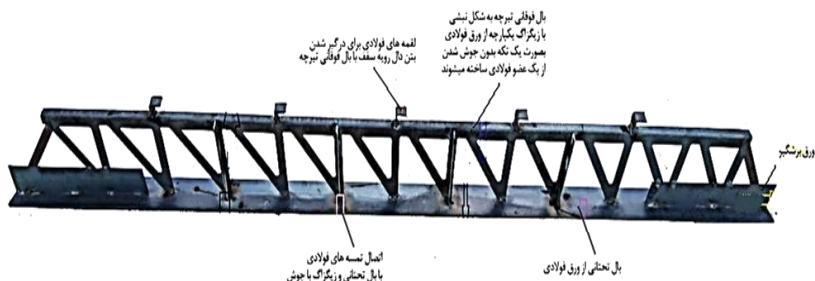
شکل ۲-۱ تیرچه یکپارچه فولادی و اجزاء آن
