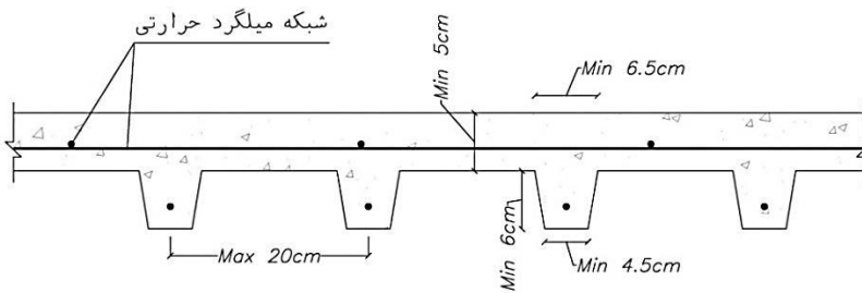
شکل ۱۲-۲ مقطع دال پس از بتن ریزی
