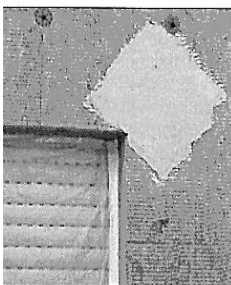
شکل ۱۳-۵ تقویت کنج‌های پنجره‌ها با یک لایه مش در زیر لایه مش اصلی
