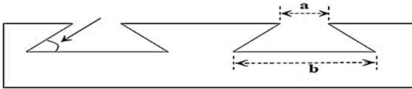
شکل ۵-۲۲ نمای کلی از پروفایل آجر دندانه‌دار؛ (زاویه منفی)
