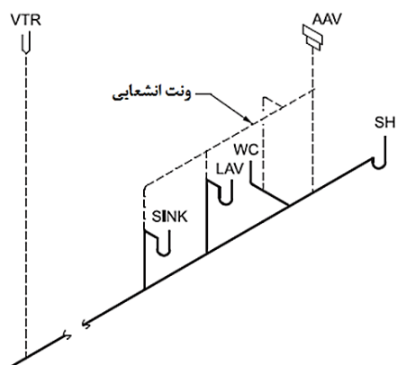
شکل ۸-۷ ونت تر
