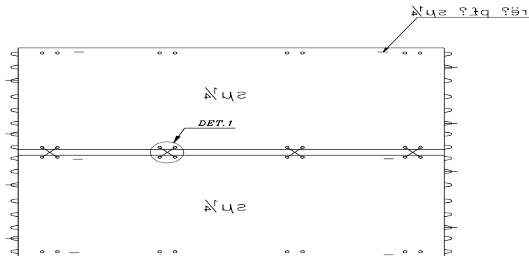
شکل ۱-۳۰ اتصال قطعات پیش‌ساخته سقف Hollow Core به یکدیگر
