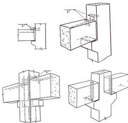
شکل ۱-۲۵ نمونه هایی از اتصالات غیر همگون با شکل پذیری محدود به صورت جوشی یا پیچ و مهره (اتصال خشک) برای اتصال تیر به کربل ستون پیش ساخته
