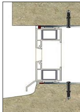
شکل ۶-۲۷ نصب پنجره کامل (همراه با شیشه) به صورت خارج از محور با بست‌های فولادی مخصوص (مطابق جزئیات ارائه شده در راهنما)
