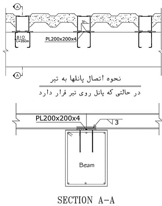
شکل ۲-۲۰ جزئیات اتصال پانل بر روی تیر بتنی
