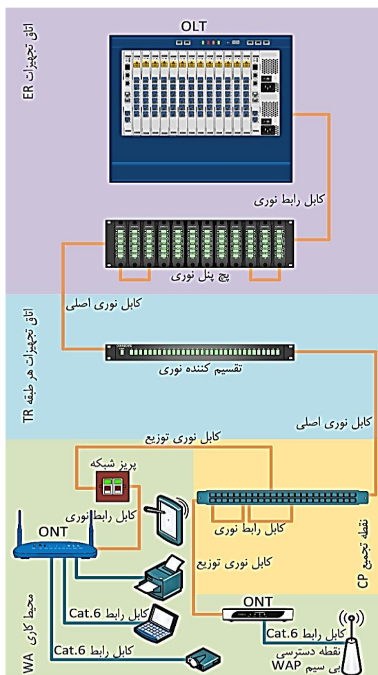
شکل ۸-۲۳- ترکیب پیچ پل فیبر
