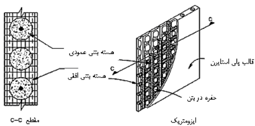
پ: قالب شبکه ای دو بعدی، حفره دار
