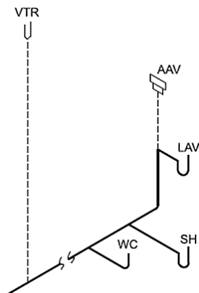
شکل ۸-۷ ونت تر
