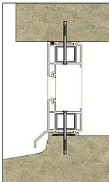
شکل ۶-۲۸ نصب قسمت‌های بازشو و شیشه‌های قسمت‌های ثابت پنجره پس از اتصال مکانیکی پروفیل پنجره به سفت کاری
