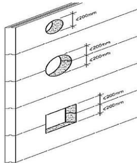
شکل ۳-۹ برش پانل برای بازشوها
