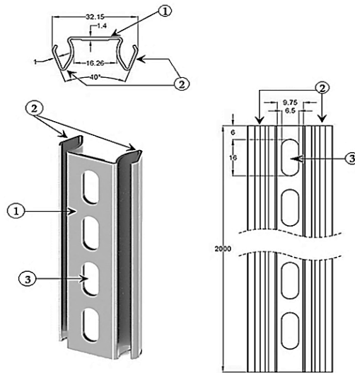
شکل ۲۴-۵ نقشه سه بعدی از پروفایل اتصال دهنده‌ی آجر نمای پلاک دندانه‌دار
