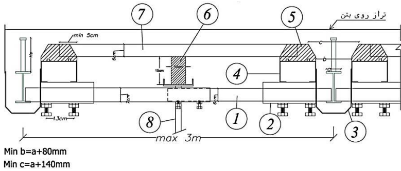
شکل ۱۱-۲ جزئیات قالب بندی
