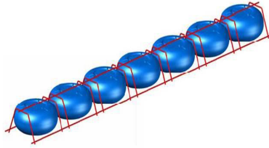
شکل ۲۷-۲- ب گوی‌های مجوف تخت برای کاهش ضخامت سقف
