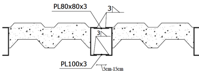
شکل ۲-۱۹ نحوه اتصال دو پانل مجاور به یکدیگر
