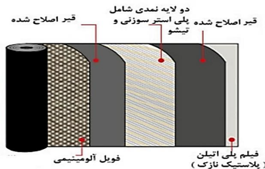
شکل ۴-۲۳ اجزای ایزوگام با قیرهای اصلاح شده
