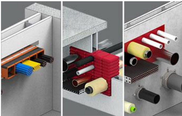
شکل ۷-۱۰ نمونه‌هایی از سیستم‌های آتش‌بند برای تأسیسات
