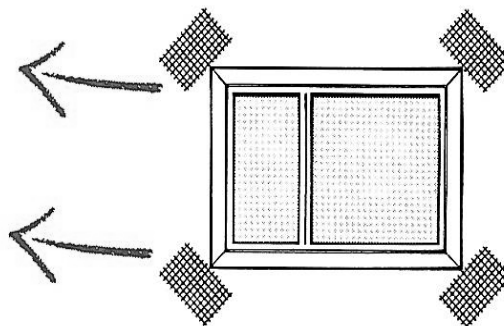
شکل ۱۳-۵ تقویت کنج‌های پنجره‌ها با یک لایه مش در زیر لایه مش اصلی
