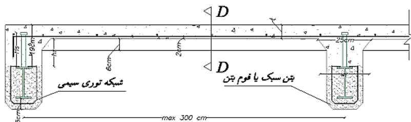
شکل ۲-۱۰ مقطع سقف کاواک
