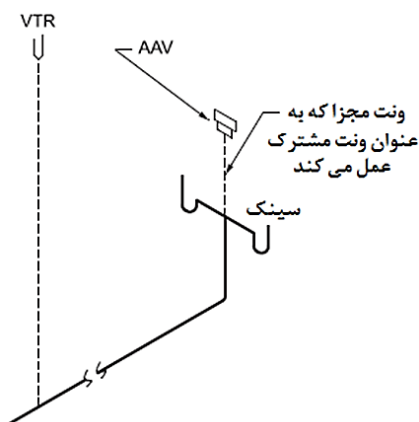
شکل ۶-۸ ونت مشترک
