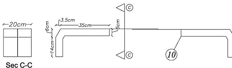
شکل ۲-۱۶ قالب میانی
