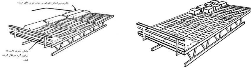
شکل ۱-۵۸ نحوه اجرای سقف‌های وافل دوطرفه و تیرچه یکطرفه با استفاده از قالب خربایی میزپرنده
