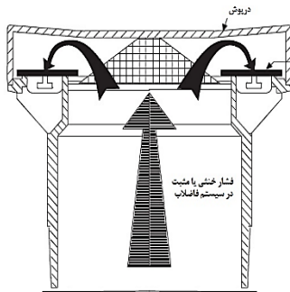
شکل ۸-۴ سوپاپ هوا گذر (AAV) در حالت بسته
