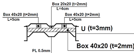
شکل ۲-۱۸ نمونه‌ای از جزئیات مقطع پانل
