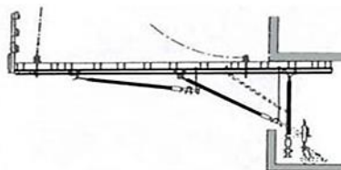
شکل ۶۲-۱ خروج قالب با حمایت کابل تاور کرین
