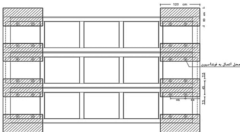
شکل ۱-۴۳ پلان موقعیت قرارگیری فونداسیون‌های پیش‌ساخته و نقاط اتصال بلوک به فونداسیون
