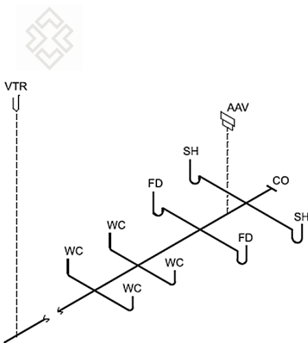
شکل ۸-۸ ونت مداری
