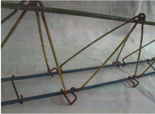
شکل ۳-۲ نمای جانبی تیرچه بدون جوش
