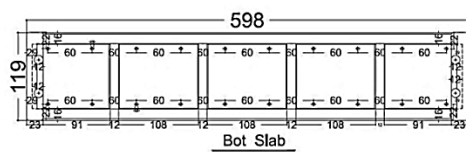
Bot Slab
