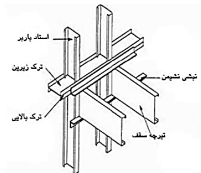
(ب) سیستم قاب بندی دیواری ممتد (Balloon Framing)
