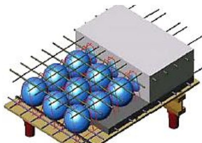
شکل ۲-۲۷-الف ساختار سقف شامل میلگردها، گوی‌ها و بتن
