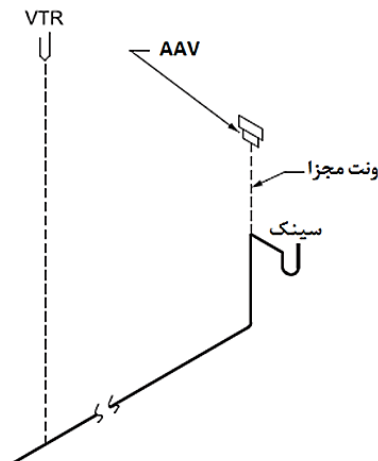
شکل ۵-۸ سوپاپ هواگذر (AAV) - ونت مجزا
