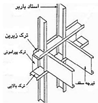
(الف) سیستم قاب بندی طبقه‌ای (Platform Framing)
