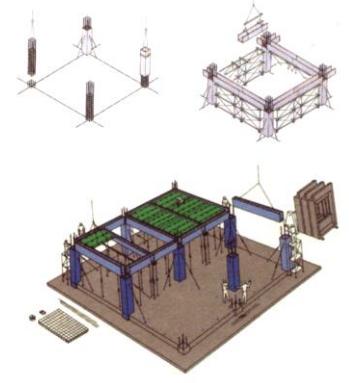
شکل ۱-۲۱ نمونه‌ای از اجرای قاب بتن مسلح پیش ساخته با ستون‌های منقطع در هر طبقه
