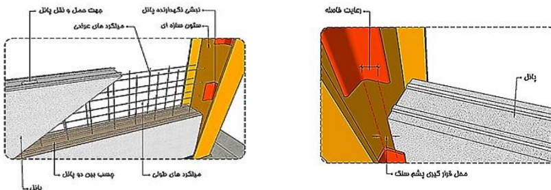
شکل ۳-۱۰ جزئیات اجرایی پانل
