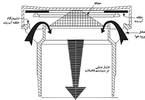
شکل ۸-۳ سوپاپ هوا گذر (AAV) در حالت باز
