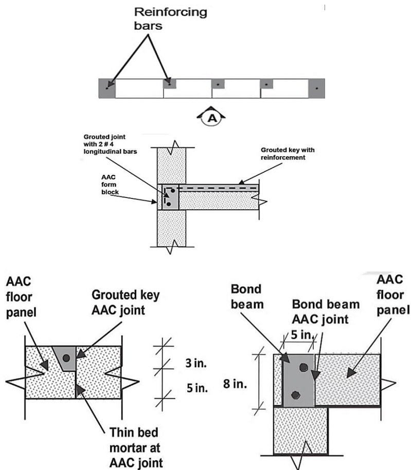
شکل ۱- ۳۷ جزئیات اجرایی اتصالات پانل
