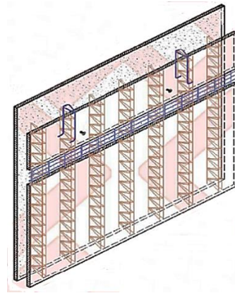
شکل ۳-۱ نمایی از پانل دیوار و تیرچه‌های قائم فولادی
