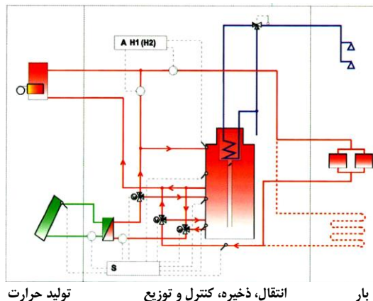
شکل ۸-۲ سیستم ترکیبی خورشیدی با کارایی بالا
