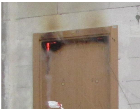
شکل ۶-۷ عملکرد ناصحیح درهای مقاوم در برابر آتش در نتیجه استفاده از مصالح ساخت نامرغوب
