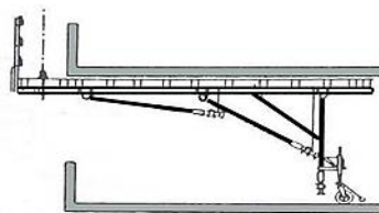
شکل ۶۱-۱ جمع شدن پایه‌ها حول مفاصل
