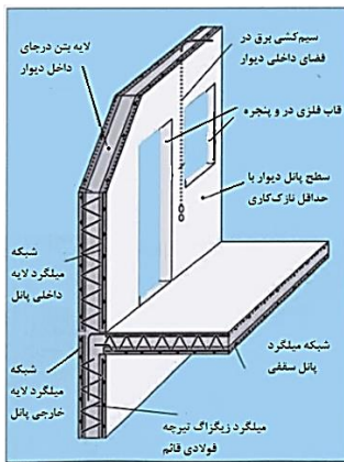
شکل ۴-۱ نمایی از سیستم دیوار دو لایه بتنی
