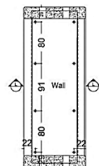
Section (WALL)
