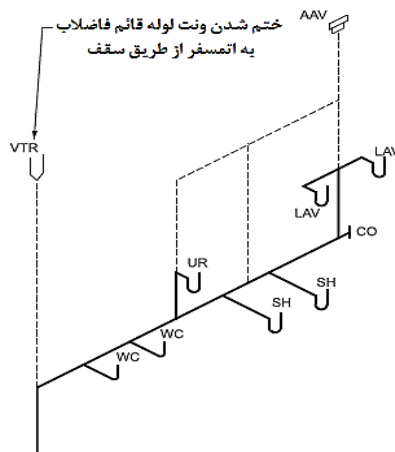
شکل ۸-۱۲ ختم شدن ونت به هوای آزاد
