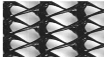
(چ) انواع ژئونت سه محوره
