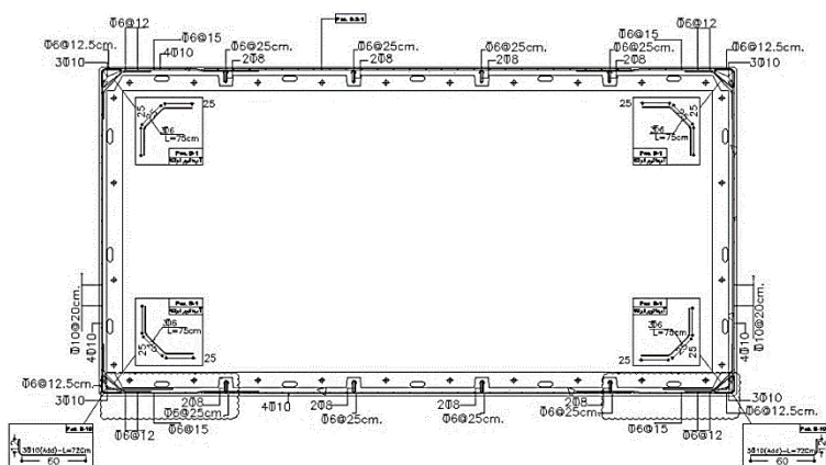
شکل ۱-۴۰ آرماتور گذاری در پوسته بلوک - مقطع طولی
