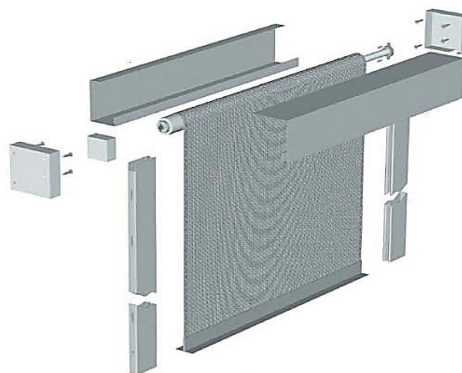
شکل ۲-۷ اجزای تشکیل دهنده پرده آتش
