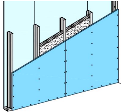
شکل ۱-۳ دیوارهای غیر سازه‌ای سبک پیش ساخته
