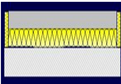
شکل ۳۵-۶ جداسازی کف شناور از دیوار به وسیله ماده الاستیک
