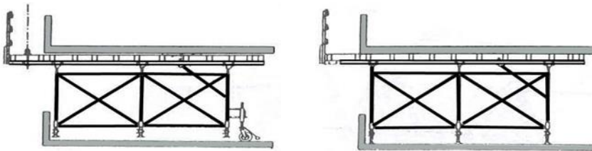
شکل ۱-۶۰ با استفاده از چرخ کمکی و جرثقیل قالب جابجا می‌شود
